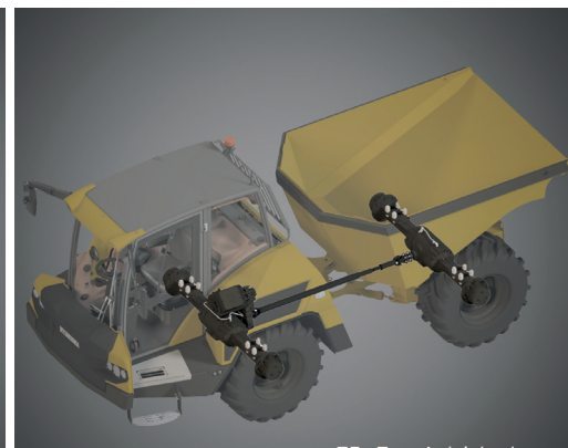
ZF eTrac Antriebsstrang
